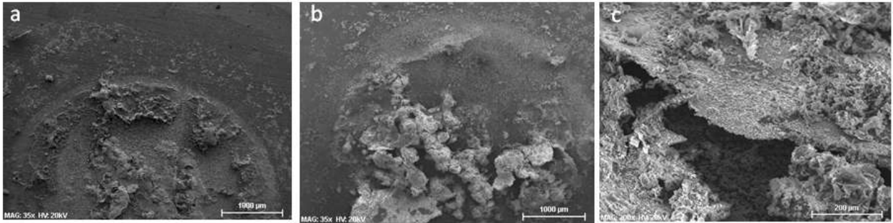
Figura 4 – MEV: a) -1,4 V 35x; b) -1,5 V 35x; c) -1,6 V 200x constante, sem agitação da solução
