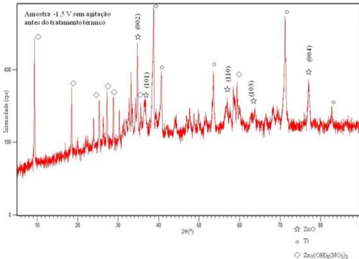
Figura 7 – Difratoograma: amostra com deposição a -1,5 V constante, sem agitação da solução
