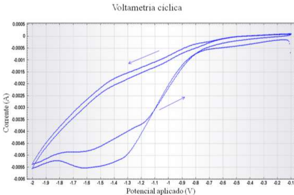
Figura 3 – Voltamograma resultante da voltametria cíclica realizada na solução de \text{Zn}(\text{NO}_3)_2 para os eletrodos utilizados
